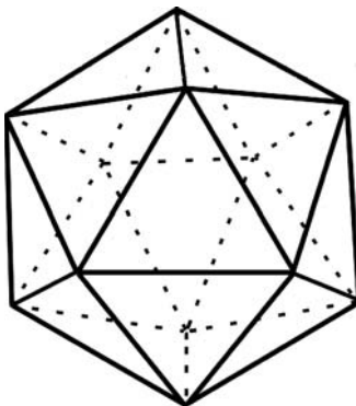
Икосаэдр
